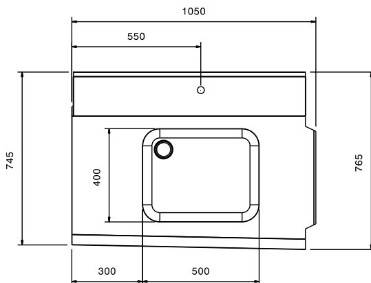
Boven aanzicht
